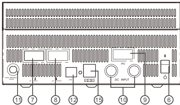
Modelos 3KVA
